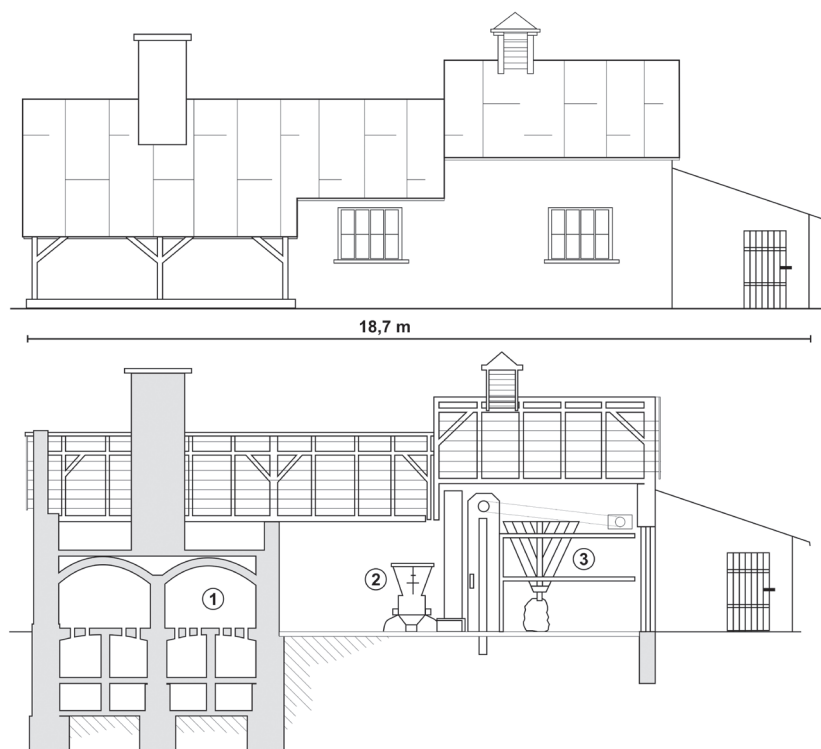
53. Gipsiarnia „Skałki” Stanisława Guzika z Bogucic. Elewacja budynku i usytuowanie urządzeń produkcyjnych na przekroju podłużnym, z oznaczeniami autora: 1 – piec komorowy, 2 – młyn do mielenia gipsu palonego, 3 – zbiornik zasypowy; według planów budowy z 1947 r. [odrysy z oryginałów]. Źródło: APK, UWK II, sygn. 21/305/0/10/2577, k. 44–46.
